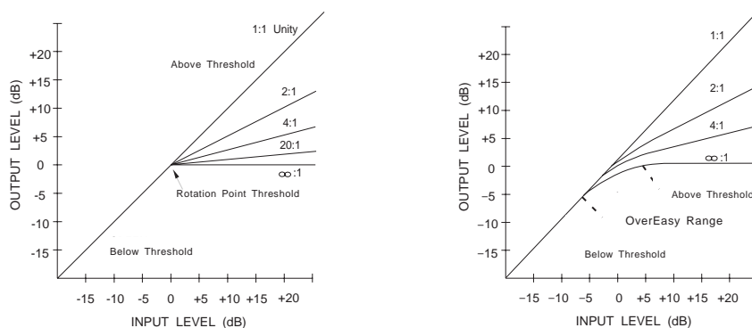
Figura 1: Curva de compresión con codo inflexible y curva de compresión OverEasy®
