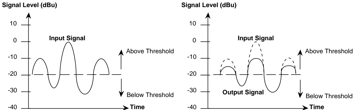
Abb. 2: Kompressionswirkung bei RATIO 2:1 und THRESHOLD bei -20 dBu
