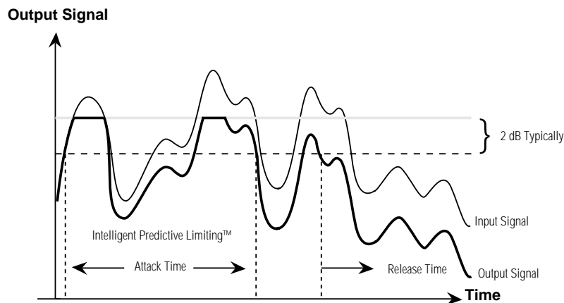
Abb. 3: Schutzfunktion des PeakStopPlus™ Limiters
