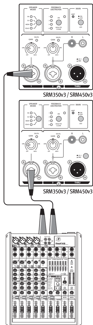
Stereo Speaker Hookup Conexión de altavoz stereo Connexion en stéréo Stereo Setup
