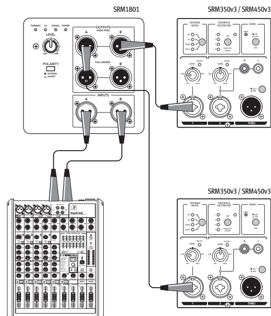
PA System with one powered subwoofer Sistema PA con un subwoofer autoamplificado Système de sonorisation avec un Subwoofer actif PA-System mit einem aktiven Subwoofer
