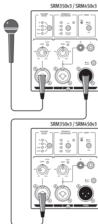
Using a microphone and daisy-chaining Uso de un micrófono y conexión en cadena Utilisation d'un micro et connexion en cascade Verwendung eines Mikrofons mit Boxen in Relhenschaltung
