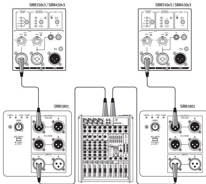
PA System with two powered subwoofers Sistema PA con dos subwoofers autoamplificados Système de sonorisation avec deux Subwoofers actifs PA-System mit zwei aktiven Subwoofern
